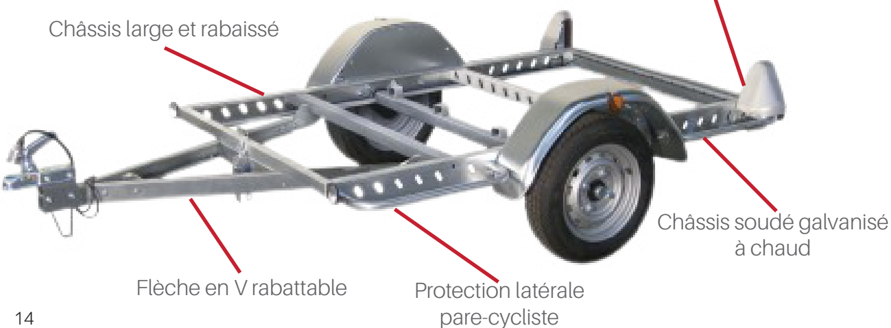
Châssis multy 115
