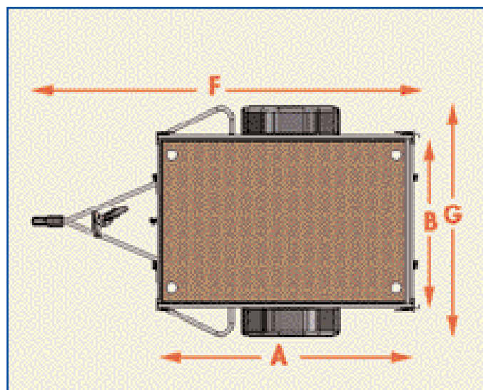
Les dimensions sont données en mètres à titre indicatif
