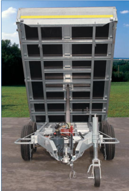
Roue jockey d'origine type TP à hauteur réglable
